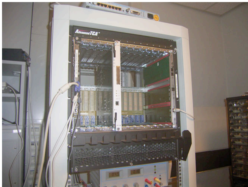
ATCA shelf と Xilinx test card
