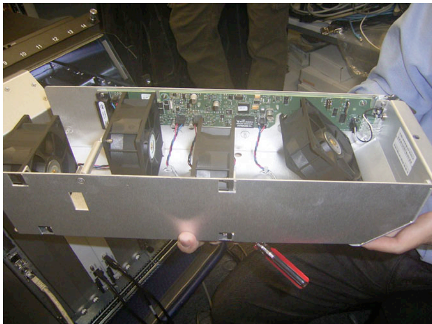
上部 Fan unit と IPMI board
