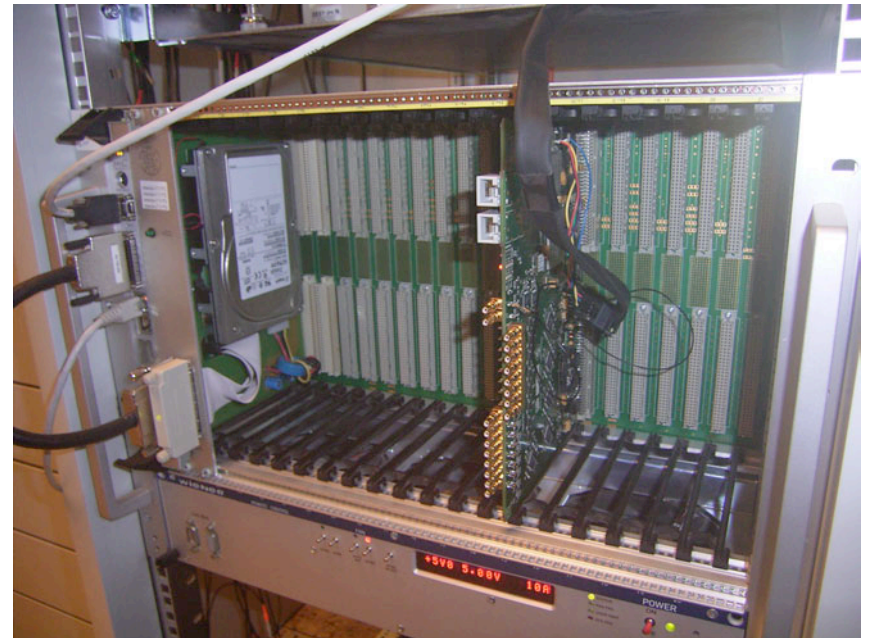
旧 VME Iirf prototype 開発
